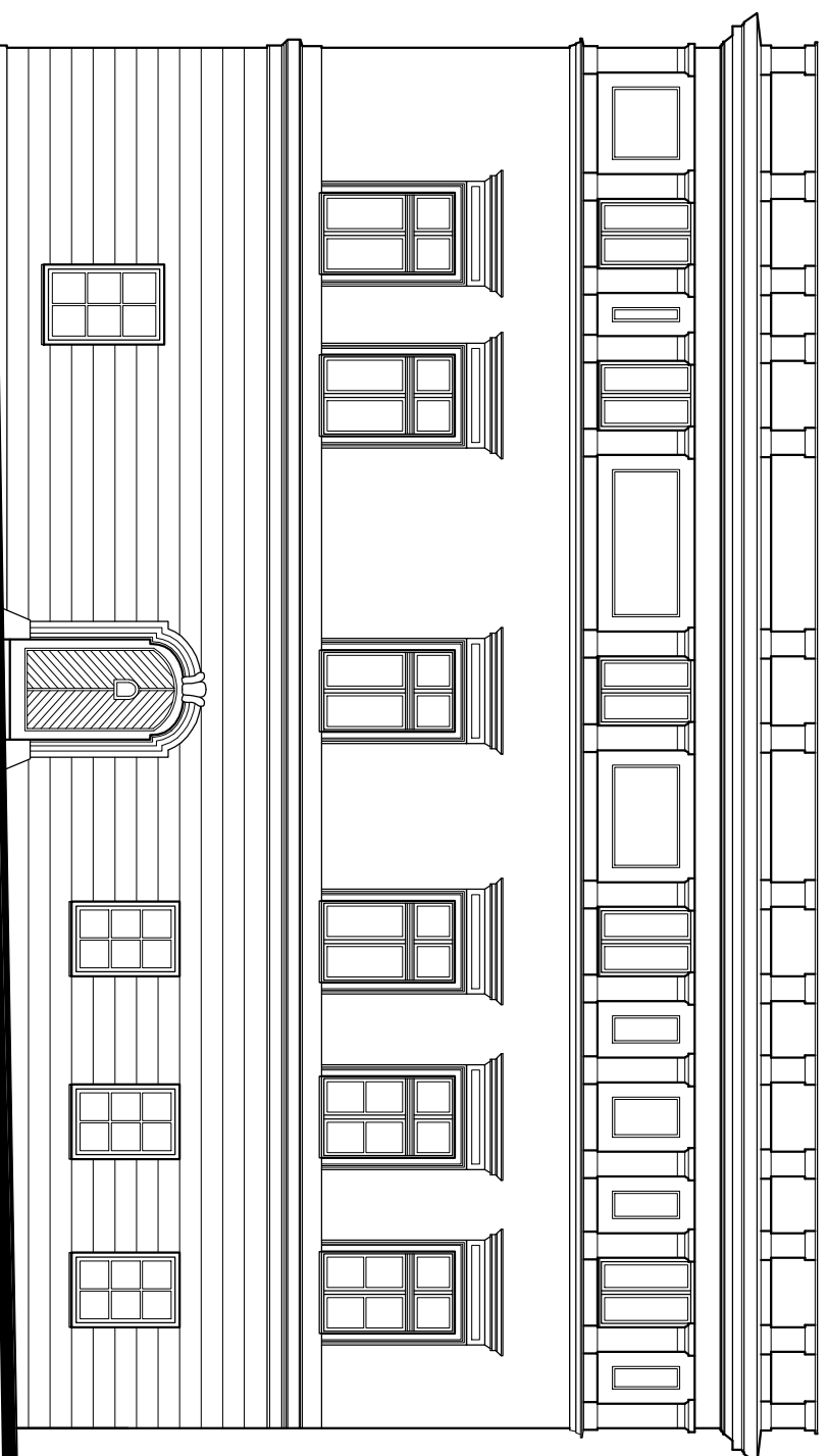
ELEWACJA POŁUDNIOWO-ZACHODNIA
